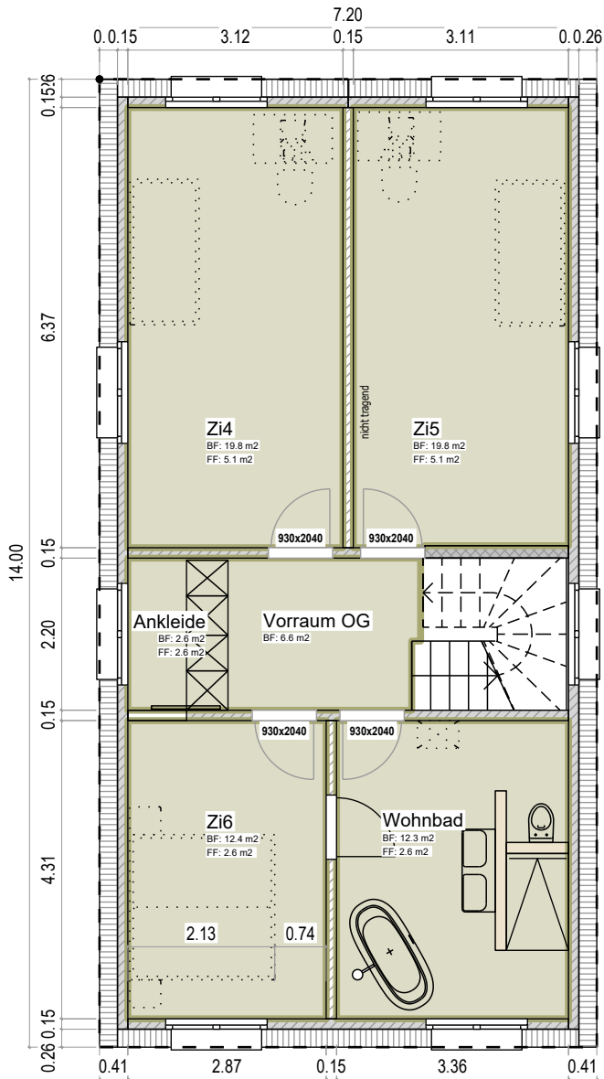
1. Dachgeschoss 1:100
