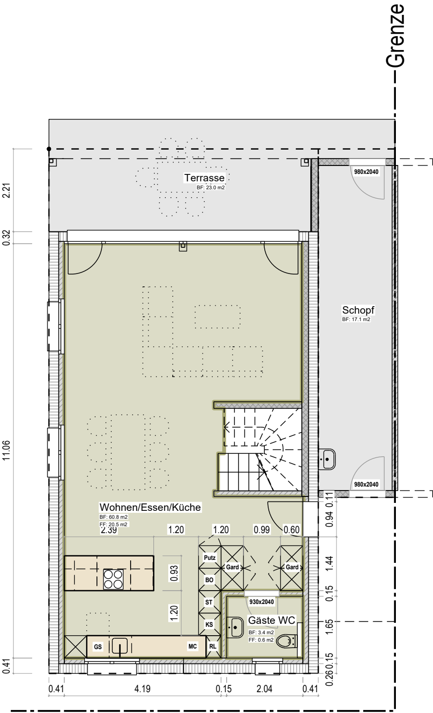
Erdgeschoss 1:100
