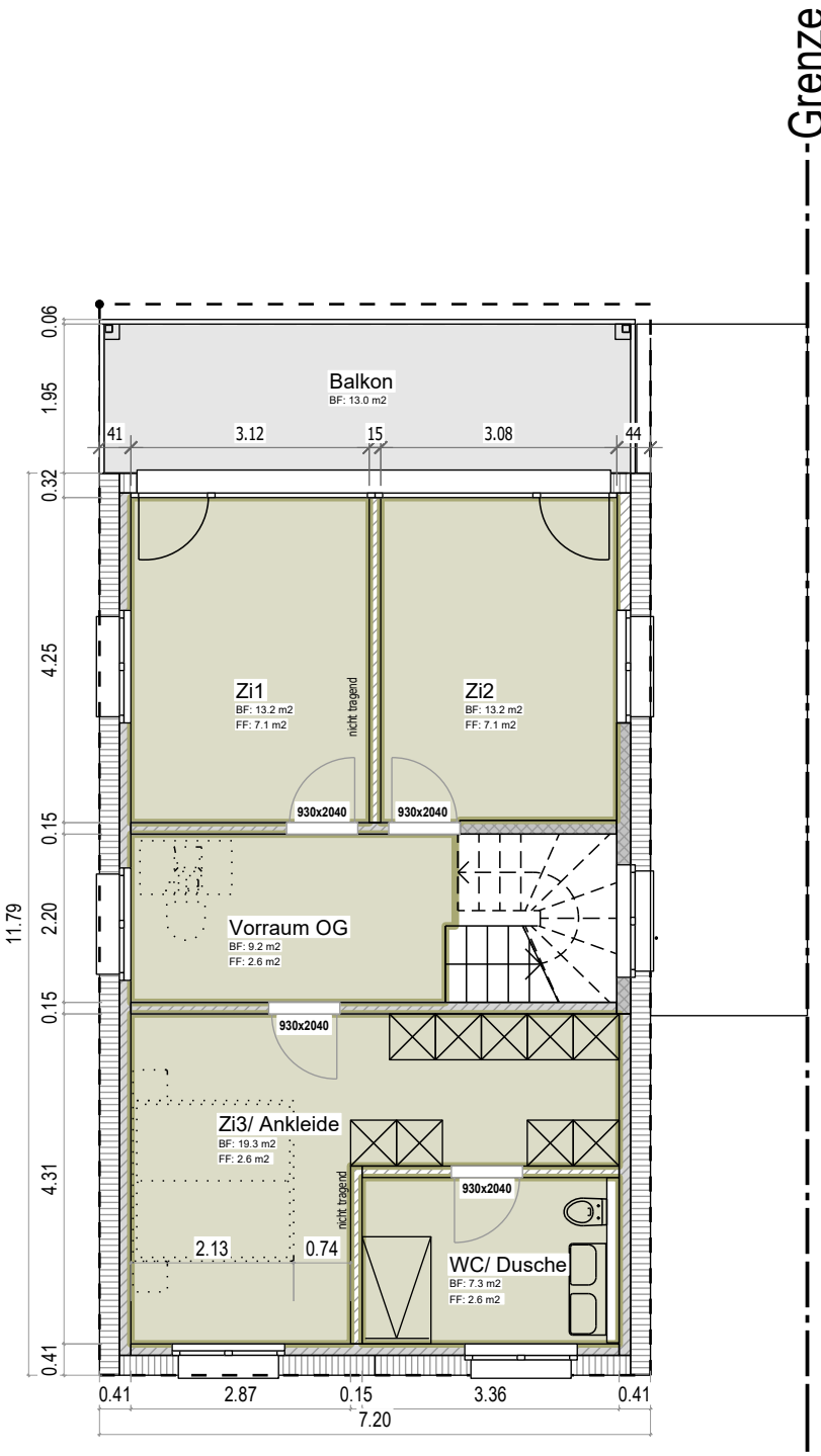
Obergeschoss 1:100
