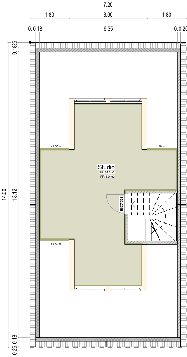
2. Dachgeschoss 1:100
